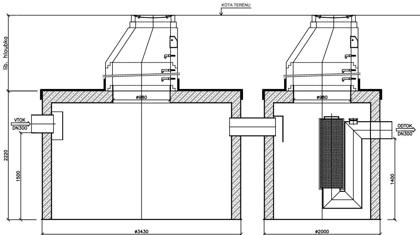
ŘEZ A-A
